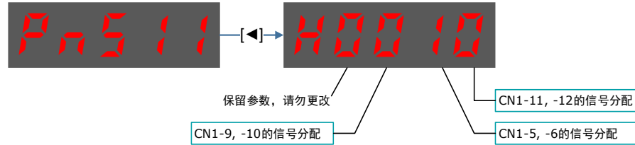
图8-3 输出信号分配示意
