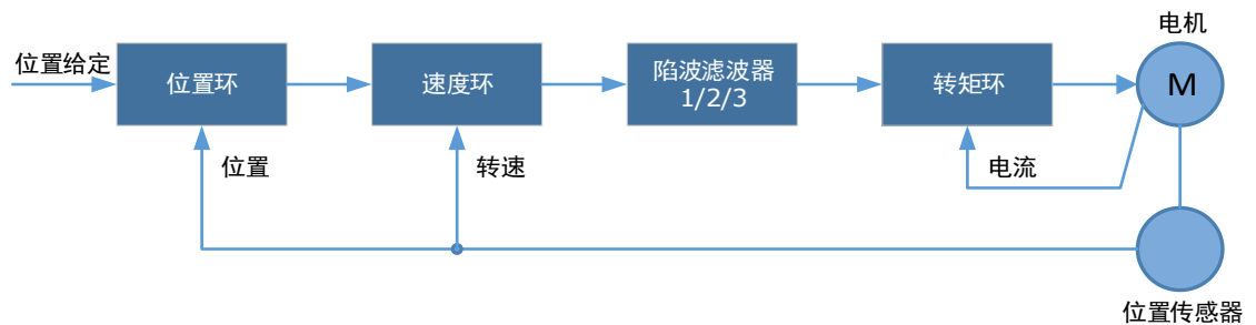
图11-30 陷波滤波器工作示意图
