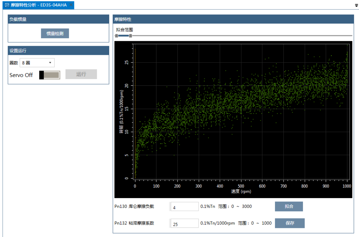
图11-59 摩擦特性的检测结果
