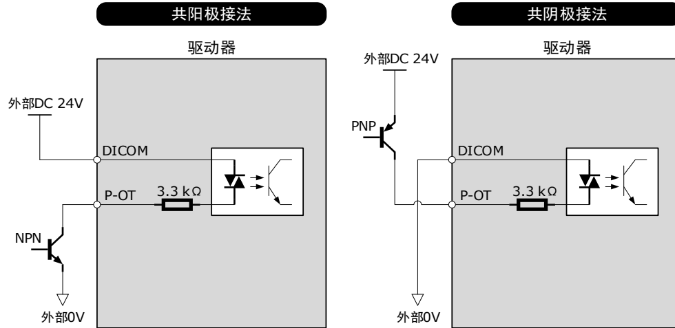
图6-3 输入信号接线示例
