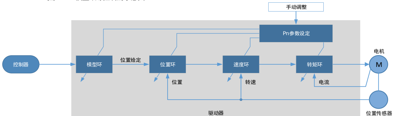
图11-29 模型跟踪控制的示意图
