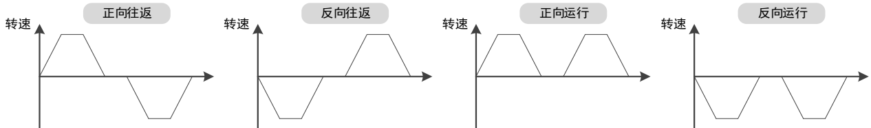
图11-9 离线自动调整时的电机运动方式
