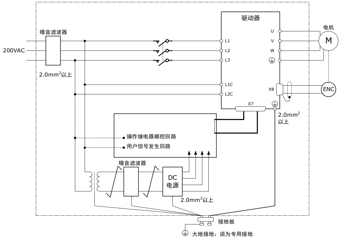
图6-1 抗干扰对策的接线示例
