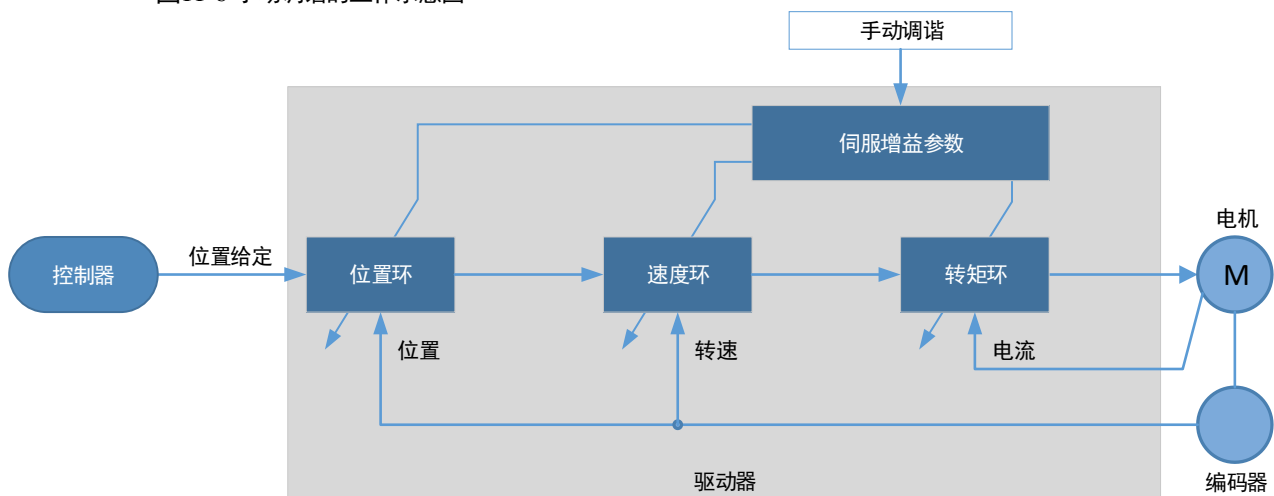
图11-6 手动调谐的工作示意图
