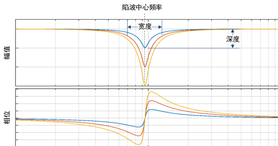
图11-31 陷波滤波器的频率特性
