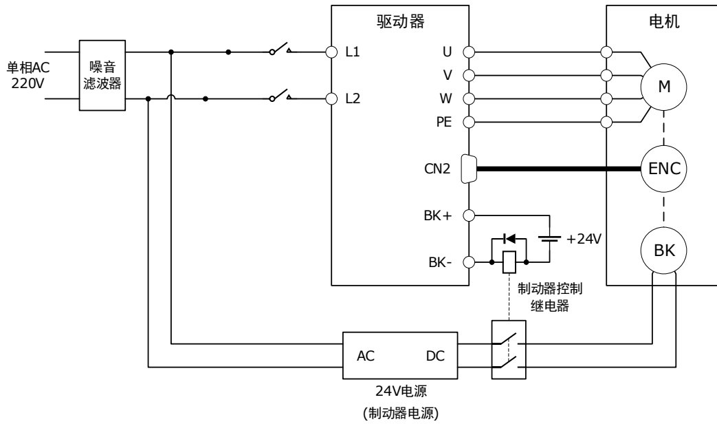
图6-6 制动器接线示例
