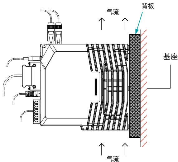
图5-1 垂直的基座安装
