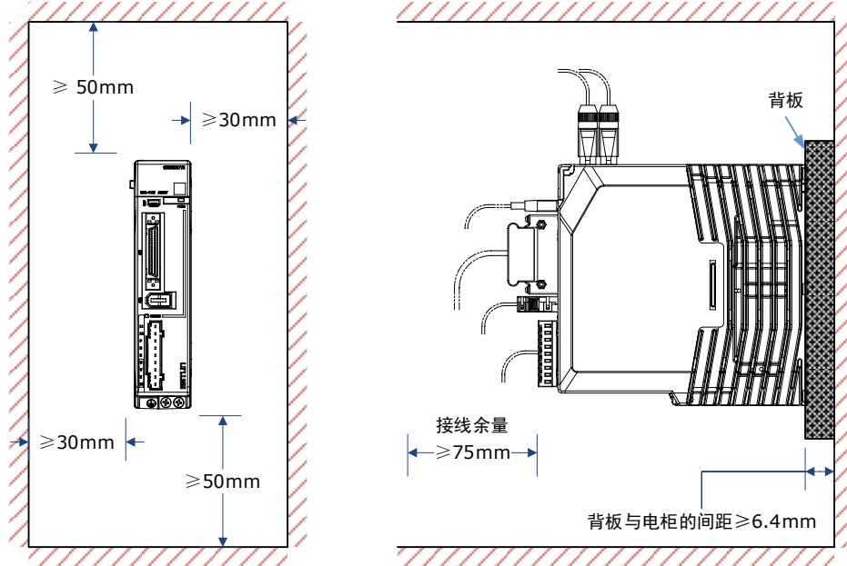
图5-2 安装单个驱动器至控制柜时
