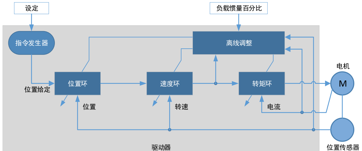
图11-7 调谐工具的工作示意图
