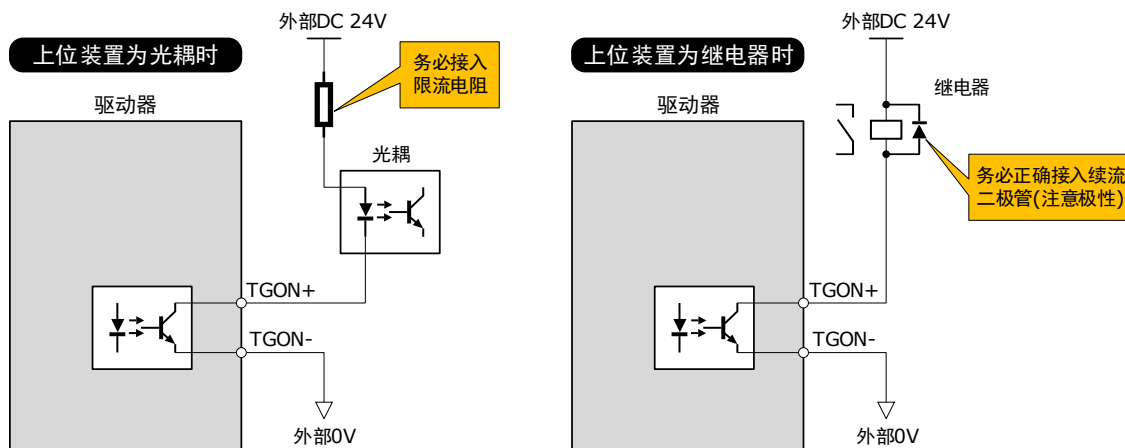
图6-4 输出信号接线示例
