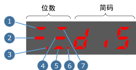
图7-3 状态显示说明
