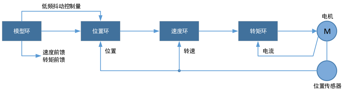
图11-34 低频振动抑制工作示意图
