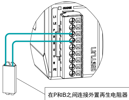
图6-2 连接外置再生电阻器示例图
