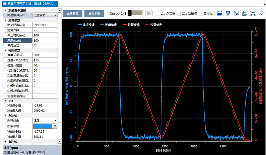
图11-21 “位置斜坡”指令采样结果的示例
