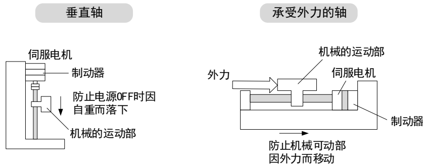
图8-2 使用制动器的场合
