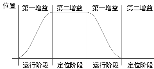
图11-23 增益切换示例
