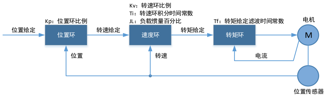
图11-2 伺服控制原理
