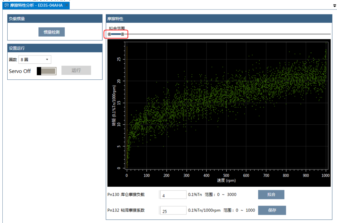
图11-60 选择拟合范围
