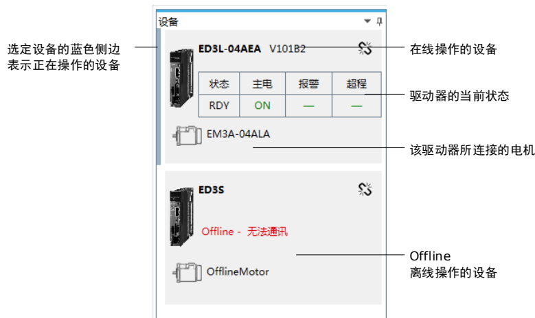
图7-34 查看设备的状态信息
