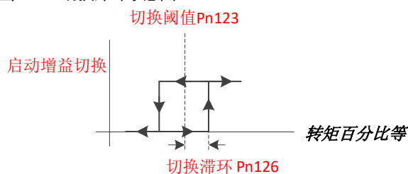
图11-25 切换滞环示意图
