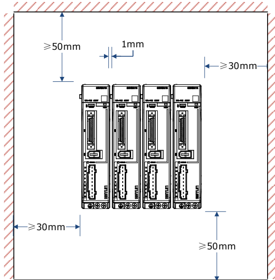
图5-3 安装多个驱动器至控制柜时
