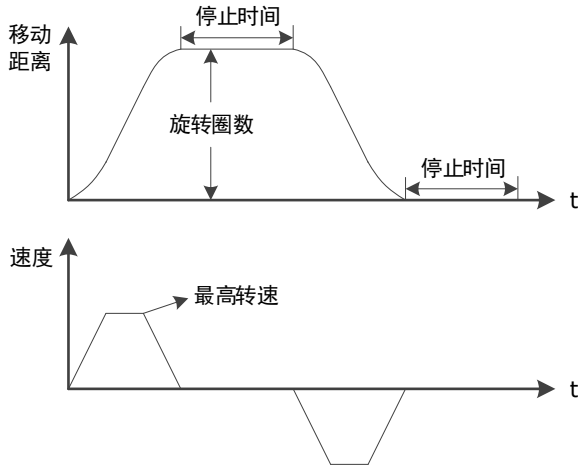
图11-8 位置节点参数
