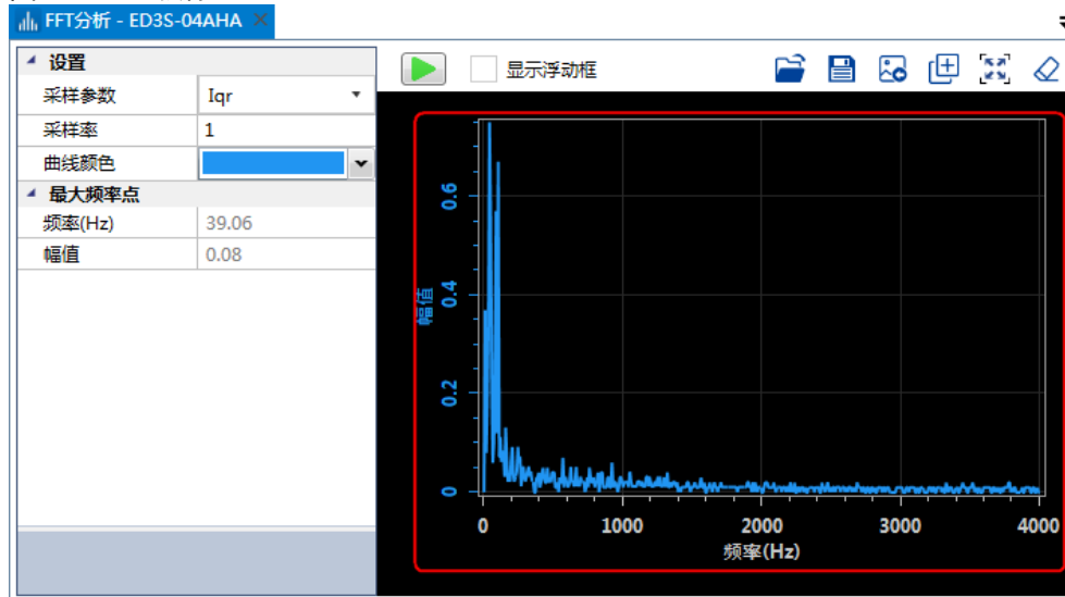
图11-52 FFT 执行结果
