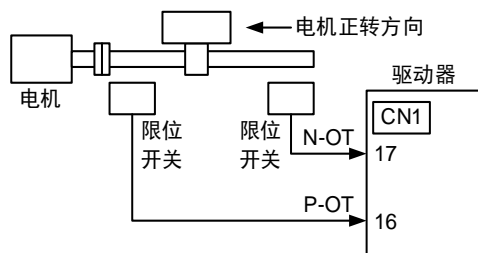
图8-1 超程信号的接线示意图
