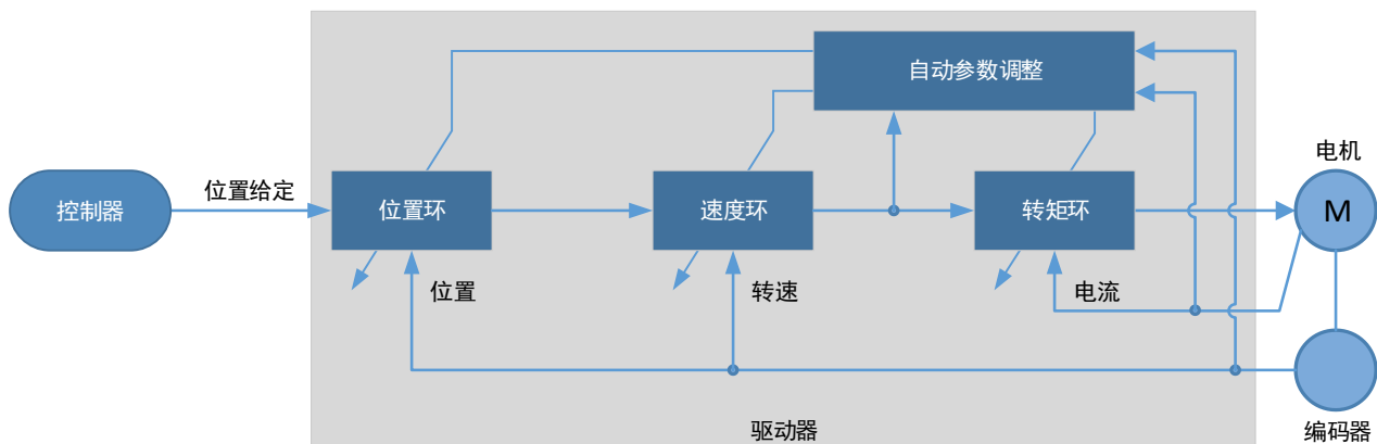
图11-4 免调谐的工作示意图
