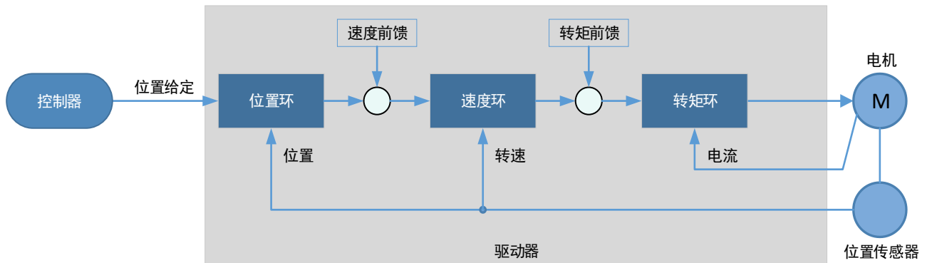
图11-26 伺服控制中的前馈示意
