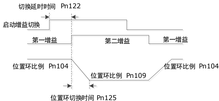
图11-24 增益切换时序图
